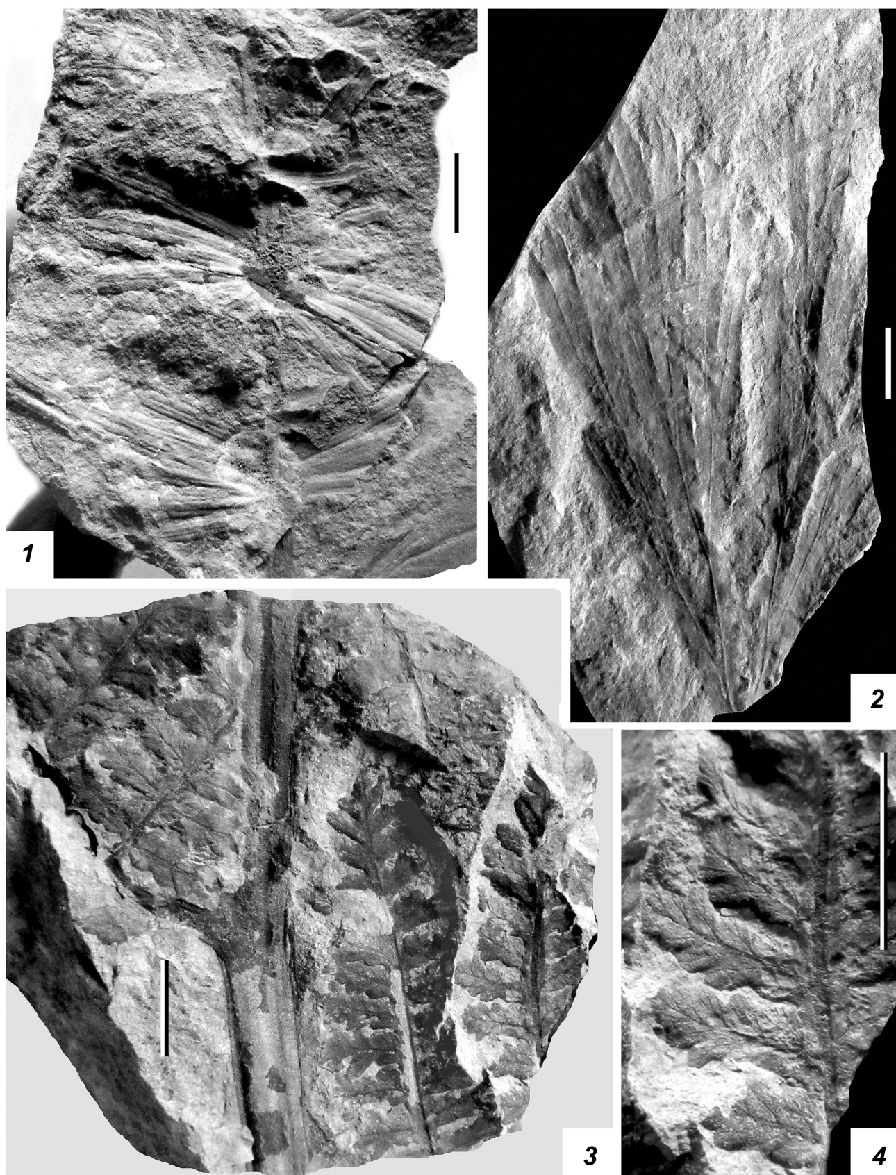
Фототабл. 4. Растительные остатки из местонахождения Воркута-1: 1 — Annulina neuburgiana (Radczenko) Neuburg, экз. МЗ ВФ 14746; часть облиственного побега; 2 — лист гинкгофита (?), экз. МЗ ВФ 14747; 3 — Pecopteris anthriscifolia (Goeppert) Zalessky, экз. МЗ ВФ 14748; средняя часть крупной вайи с тремя порядками сегментации; 4 — P. anthriscifolia (Goeppert) Zalessky, строение пера последнего порядка экземпляра (3). Длина масштабной линейки 1 см
