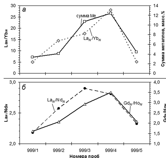
Рис. 2. Сопоставление распределения рудных элементов с характеристиками спектров РЗЭ в пробах по разрезу через жилу Гацировская: а — изменение суммарного содержания металлов ( \Sigma \text{Me} = \text{Fe} + \text{Zn} + \text{Pb} + \text{Cu} ) и отношения \text{La}_N:\text{Yb}_N ; б — изменение отношений \text{La}_N:\text{Nd}_N и \text{Gd}_N:\text{Ho}_N по разрезу
