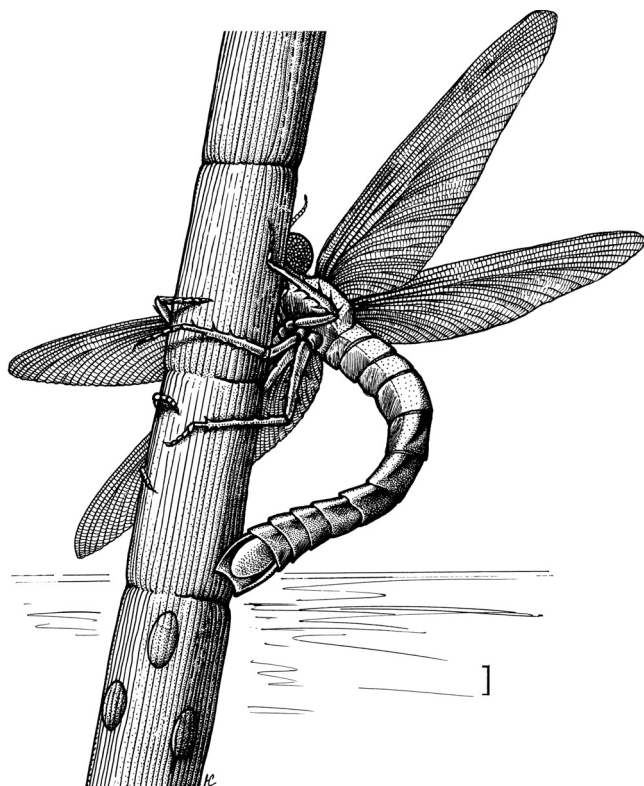
Рис. 3. Гигантская пермская стрекоза-меганеврида Arctotypus sylvaensis Martynov формирует яйцекладки на побеге крупного хвощевидного. Длина масштабной линейки 1 см
