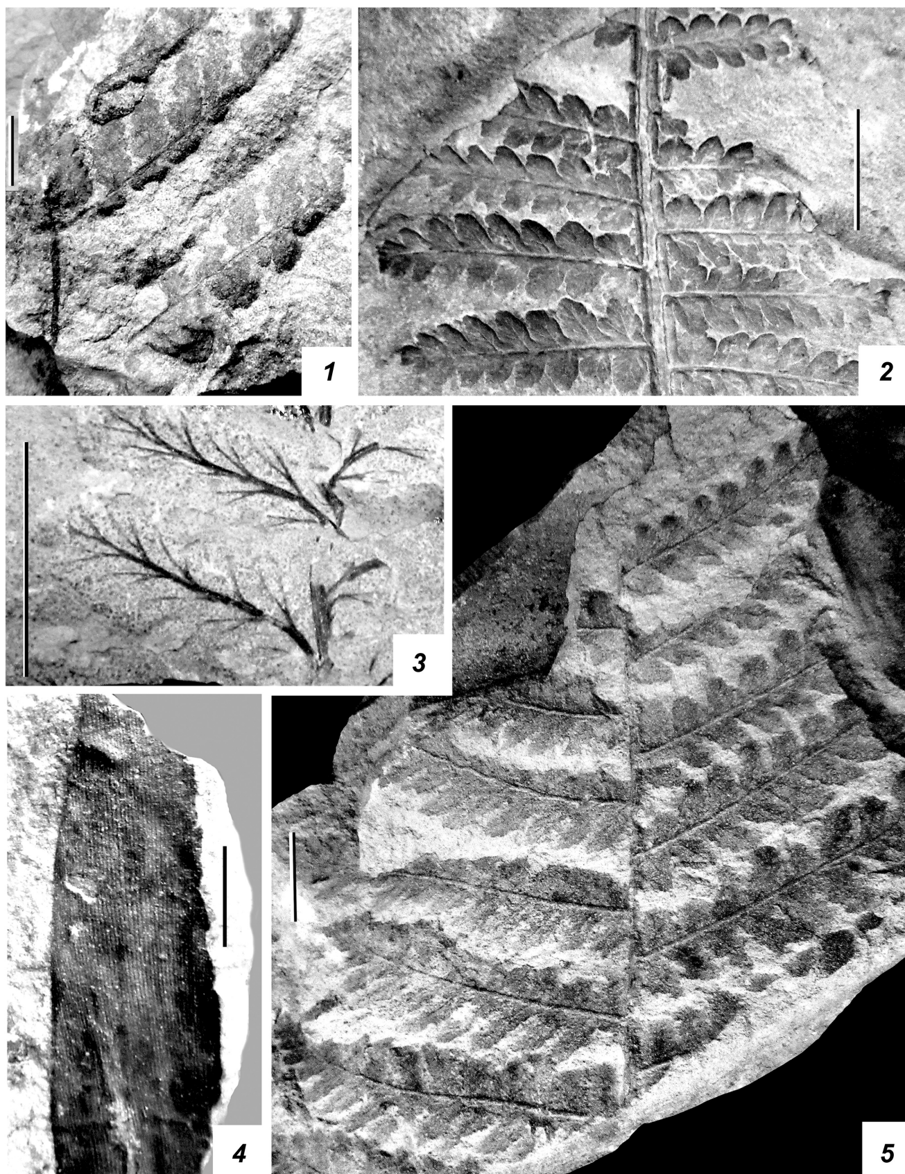
Фототабл. 3. Растительные остатки из местонахождения Воркута-1: 1 — Pecopteris anthriscifolia (Goeppert) Zalessky, экз. МЗ ВФ 14744; средняя часть вайи с двумя сохранившимися перьями последнего порядка; 2 — P. cf. leptophylla Bunbury, экз. МЗ ВФ 14741; средняя часть вайи (перо предпоследнего порядка); 3 — P. helenaeana Zalessky, экз. МЗ ВФ 14738; два стерильных перышка (сегменты последнего порядка); 4 — Ruf flora sp., экз. МЗ ВФ 14745; фрагмент ланцетовидного листа голосеменного порядка войновские (Vojnovskyales); 5 — Pecopteris anthriscifolia (Goeppert) Zalessky, экз. МЗ ВФ 14739; приапикальная часть вайи. Длина масштабной линейки 1 см
