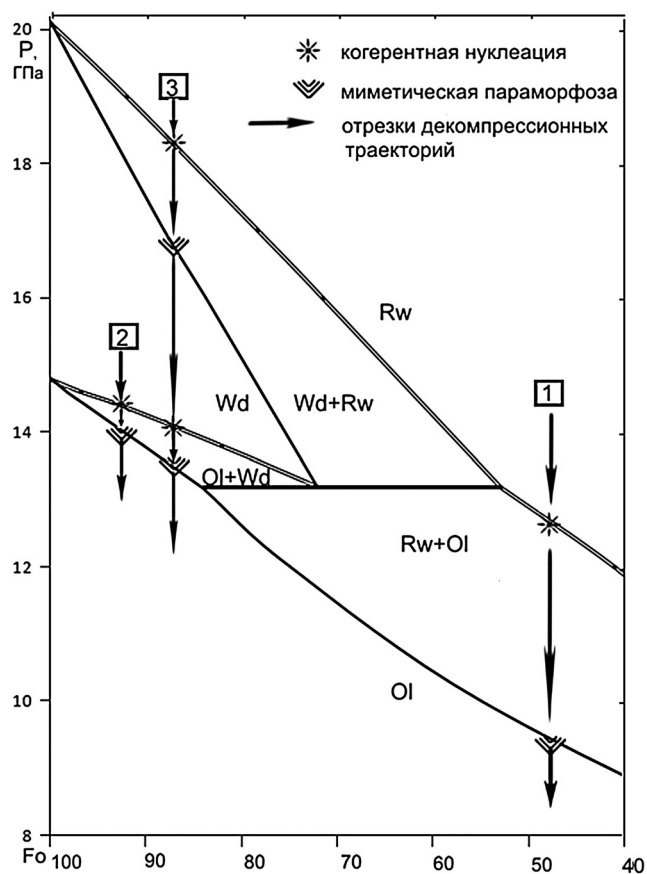
Рис. 1. Изотермическое ( T=1873 К) сечение магнезиальной части фазовой диаграммы системы (\text{Mg,Fe})_2\text{SiO}_4 , по [Akaogi et al., 1989], с декомпрессионными траекториями
