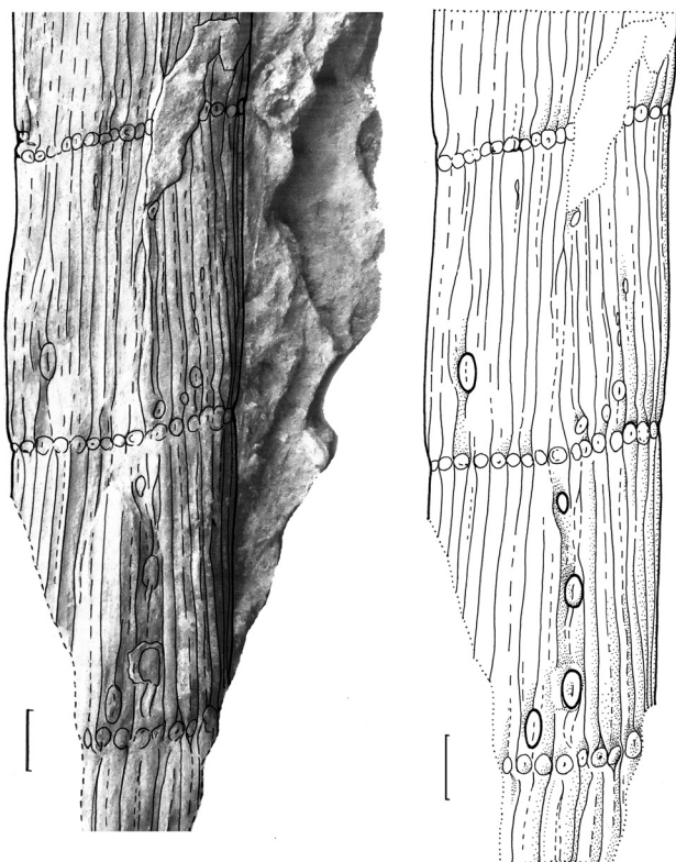
Рис. 2. Побег хвощевидного Paracalamitina cf. striata Zalesky emend. Naug. с предполагаемыми яйцекладками стрекоз, экз. МЗ ВФ 14743. Слева — графическое дешифрирование морфологии побега; справа — прорисовка. Длина масштабной линейки 1 см
