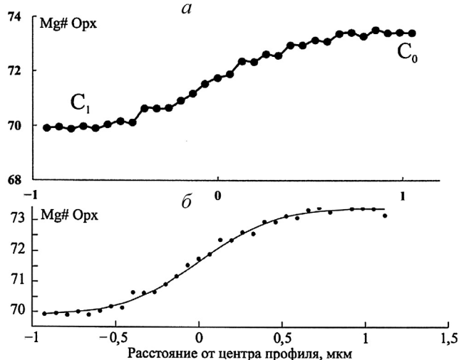
Рис. 1. Фото вкрапленника ортопироксена с обратной зональностью. Образец BZ-10-4, фото в отраженных электронах вверх; белые линии — направления, по которым построен профиль (а), и с помощью программы ImageJ аппроксимированный в программе DataFit профиль (б) по линии а (на фото)
