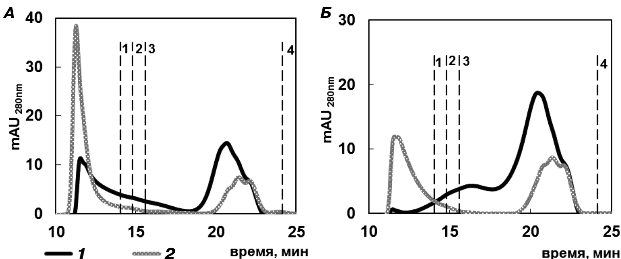
Рис. 3. Хроматограммы распределения органических веществ исследуемых почвенных (А) и болотных (Б) вод: 1 — до облучения, 2 — после облучения. Прерывистыми вертикальными линиями нанесены стандарты («Dalton Standards MS-II», SERVA): 1 — химотрипсिनоген (25,0 кДа), 2 — миоглобин (17,8 кДа), 3 — цитохром С (12,3 кДа), 4 — DNP-L-аланин (255,2 Да)
