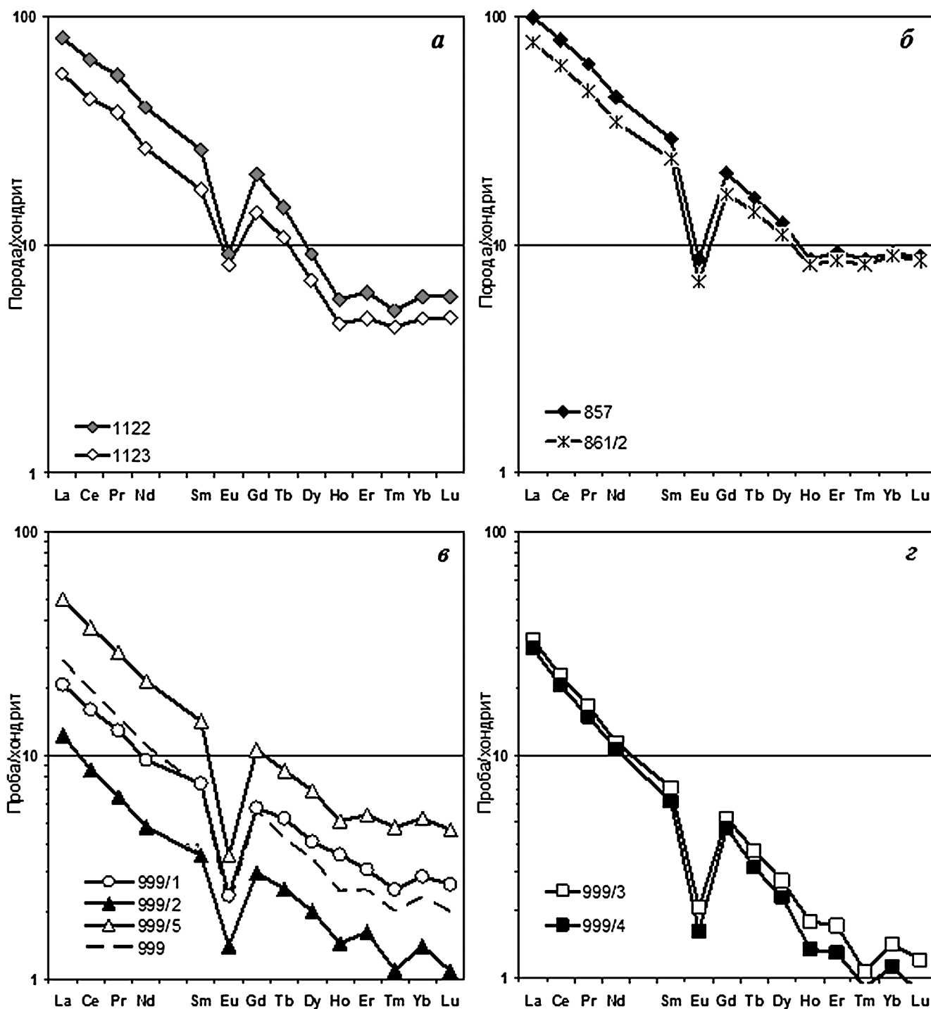
Рис. 1. Нормированное на хондрит, по [Palme&Jones, 2003], содержание РЗЭ во вмещающих породах и в рудных пробах по разрезу через жилу Гашировская (месторождение Верхнезигидское): а — спектры палеозойских гранитов на расстоянии от жилы 50 и 100 м (№ 1122, 1123); б — спектры околожильных пород на расстоянии от жилы 150 и 240 см (№ 857, 861/2); в — спектры проб из приконтактных частей жилы (№ 999/1, 999/2, 999/5) и сборной пробы (№ 999); з — спектры проб из центральных частей жилы (№ 999/3, 999/4)
