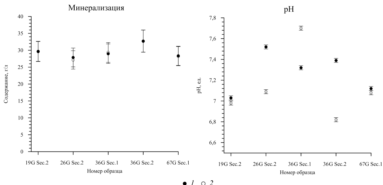
Рис. 5. Значения минерализации и величины pH поровых вод, измеренные (1) и рассчитанные (2) по данным водных вытяжек с учетом естественной влажности отложений
