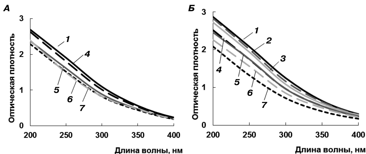
Рис. 2. Изменение значений оптической плотности почвенных (А) и болотных вод (Б) в ходе экспериментов: 1 — нулевой день, 2 — первый день, 3 — второй день, 4 — третий день, 5 — четвертый день, 6 — пятый день, 7 — десятый день
