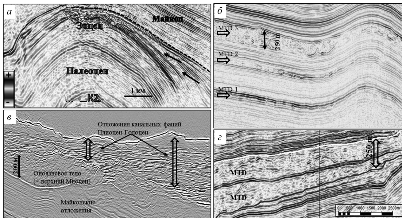
Рис. 5. Фрагменты сейсмических разрезов: а — строение отложений палеоцена—эоцена в районе Анапского выступа; б — отложения MTD в Туапсинском прогибе; в — район современного континентального склона Черного моря; г — отложения MTD в районе Анапского выступа
