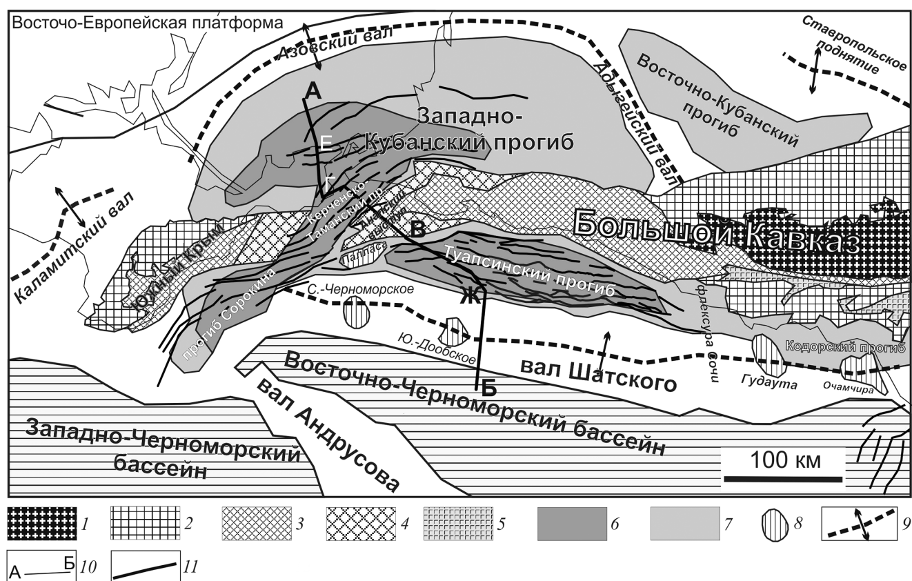
Рис. 1. Тектоническая схема Восточно-Черноморского региона и прилегающих территорий (составлена с учетом данных [Афанасенков и др., 2007; Митюков и др., 2012; Nikishin et al., 2015a, b; Okay et al., 1997, 2003]: 1 — докембрийские кристаллические массивы; 2 — орогены, сложенные шельфовыми осадочными породами мезозоя-эоцена; 3 — орогены, сложенные мезозойско-эоценовыми глубоководными отложениями; 4 — части орогенов, перекрытые майкопско-четвертичными отложениями; 5 — мезозойские вулканиты; 6 — депозиты олигоцен-современных молассовых бассейнов с толщиной майкопских отложений более 4–5 км; 7 — неглубокие олигоцен-современные молассовые бассейны; 8 — кайнозойские тектонические поднятия; 9 — оси поднятий, активных в олигоцене; 10 — положение композитного профиля А-Б; 11 — взбросо-надвиговые нарушения в олигоцен-миоценовых отложениях
