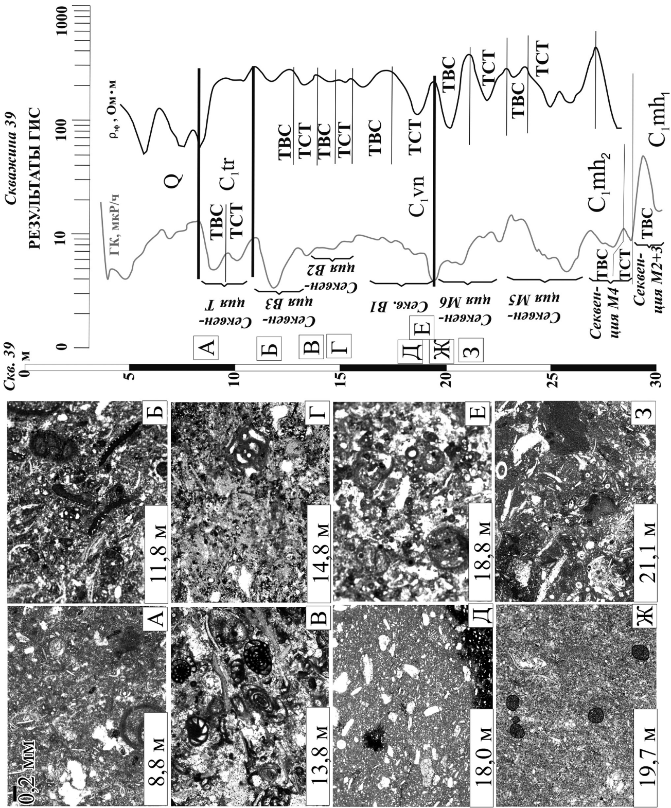
Рис. 5. Петрографическая и геофизическая характеристика разреза визейско-серпуховских отложений в скважине № 39. Слева фото шлифов в проходящем свете: интервал 8,30–12,40 м, тарусский горизонт: А — образец (обр.) 39/8,8 м, пакстоун, известняк биоморфный; В–Е — интервал 12,40–20,0 м, веневский горизонт: В — обр. 39/13,8 м, грейнстоун, известняк с биокластами; Г — обр. 39/14,2 м, грейнстоун, известняк биоморфный; Д — обр. 39/18,0 м, пакстоун, известняк с биокластами; Е — обр. 39/18,8 м, грейнстоун, известняк биоморфный; Ж–З — интервал 20,40–29,50 м, михайловский горизонт: Ж — обр. 39/19,7 м, пакстоун, известняк с биокластами; З — обр. 39/21,1 м, пакстоун, известняк биоморфный, интервал 33,2–40,0 м. Справа — результаты ГИС (гамма-картаж, мкР/ч и удельное сопротивление (Ом·м)). Буками показано положение образцов в разрезе скважины
