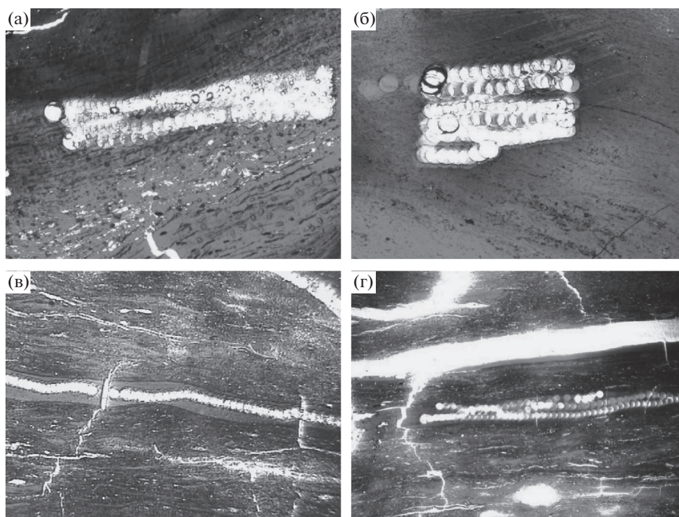
Рис. 3. Мацералы углей и точки зондирования (следы лазерного микроотборника): проба Пн-9 — структурный древесинный разложенный витринит (а); проба Пн-6 — слабоструктурный витринит из пробы угля с концентрацией германия 429 г/т в угле (б); проба Пн-3 — прослой теловитринита, в центре, с цепью точек лазерного микроанализа (из пробы угля с концентрацией германия 1290 г/т в угле) (в); проба Пн-3 — липоидо-аттрито-гелит со слоями точек лазерного микроанализа (г). Шлиф. Проходящий свет. Увеличение 100.
