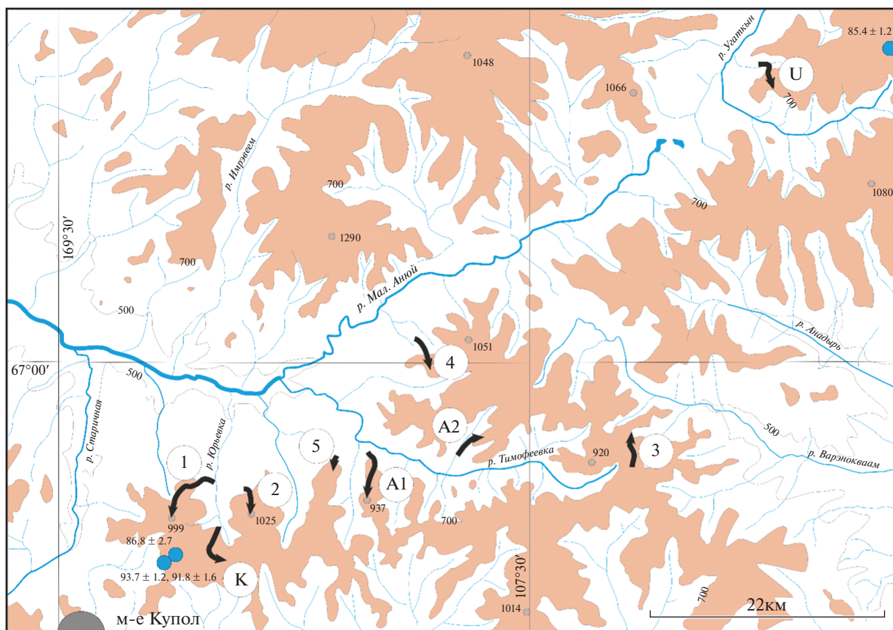
Рис. 2. Схема расположения изученных разрезов в районе месторождения Купол. Разрезы: U — Угаткын; K — Купол, г. Коваленко; A1 — Анюй 1, г. Кайемнай; A2 — Анюй 2, г. Тимоевская; 1 — г. Белая; 2 — р. Юрьевка; 3 — верховья р. Тимоевская; 4 — р. Анюй; 5 — р. Ветвистый; голубыми кружками отмечено местоположение отбора проб для ближайших изотопных датировок, обсуждаемых в тексте и их значение возраста.
