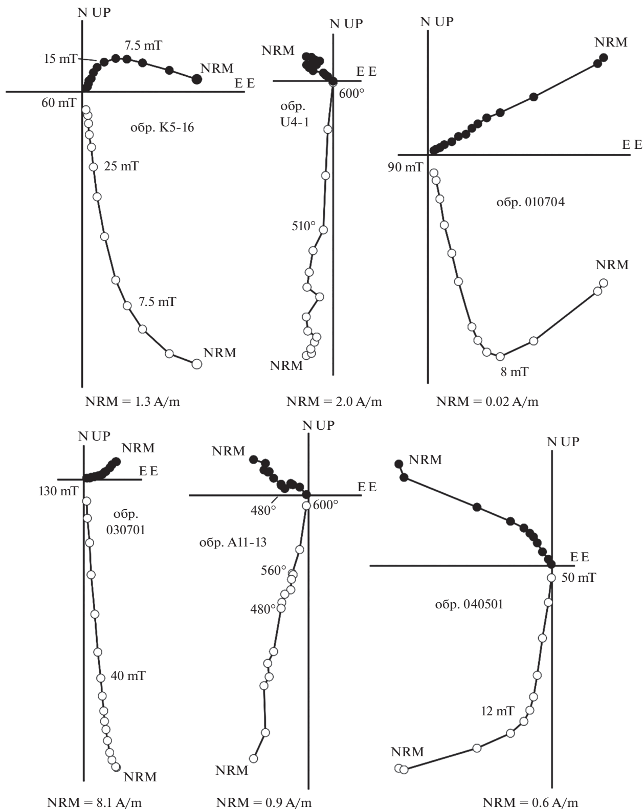
Рис. 3. Примеры диаграмм Зийдерведа по результатам магнитных чисток пород из разрезов К (обр. K5-16), У (обр. U4-1), 01 (обр. 010704), 03 (обр. 030701), А1 (обр. А11-13), 04 (обр. 040501). Черные (белые) кружки обозначают проекции вектора естественной остаточной намагниченности на горизонтальную (вертикальную) плоскость.
