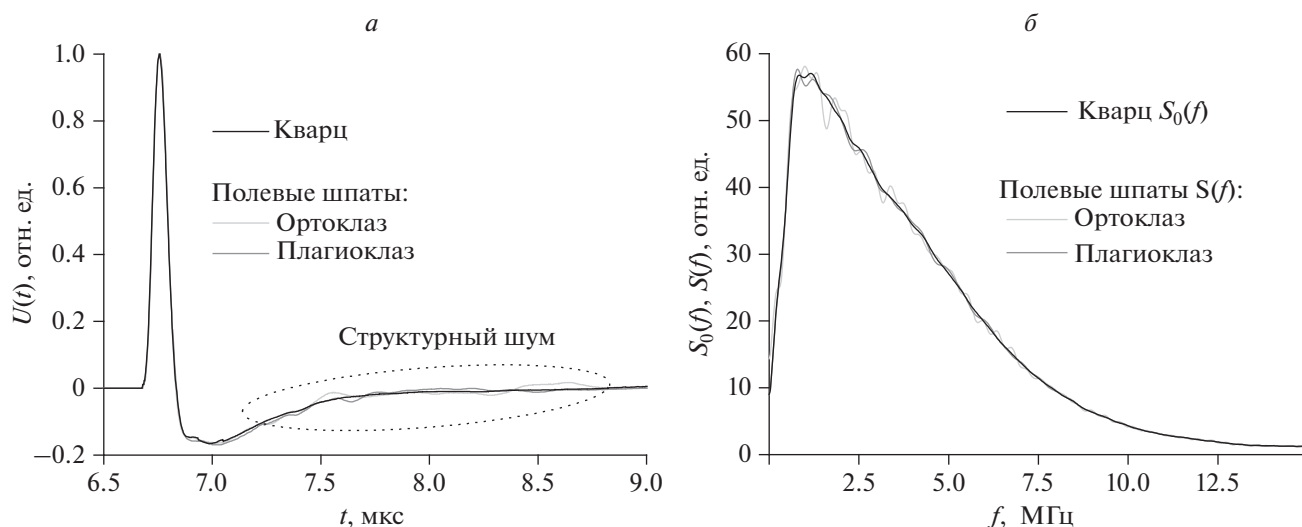
Рис. 3. Примеры ультразвуковых сигналов от кварцевой пластины и образцов ортоклаза (участок 3) и плаггиоклаза (участок 4): временные профили (а) и соответствующие спектры (б).
