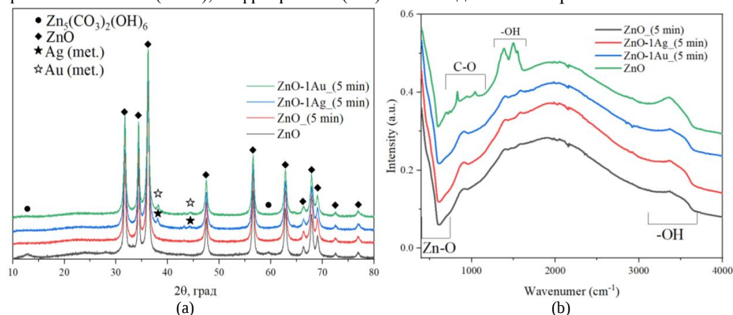
Рис. 1. Рентгенограммы (a) и ИК-спектры синтезированных образцов (b)
