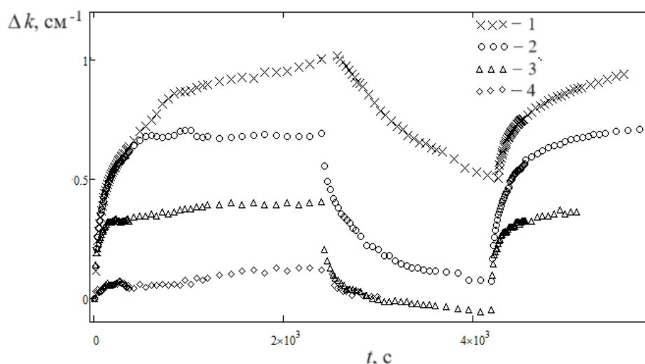
Рис. 1. Динамика изменения показателя поглощения света в кристалле \text{Bi}_{12}\text{TiO}_{20}\text{:Zn,P} на длине волны 532 нм при температуре: 1 – 23, 2 – 40, 3 – 45, 4 – 53 °C
