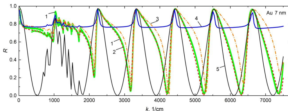
Рис. 2. Коэффициент отражения слоистой структуры №2 в зависимости от волнового числа. Эксперимент (1), расчет (2–5): 2 – R_{S0}=25\text{ Ом}/\Omega , \tau=5 фс, p=0,94 , g=0,68 ; 3 – R_{S0}=25\text{ Ом}/\Omega , \tau=5 фс, p=1,0 ; 4 – R_{S0}=25\text{ Ом}/\Omega , \tau=0 фс, p=1,0 ; 5 – R_{S0}=377\text{ Ом}/\Omega , \tau=0 фс, p=1,0 .
