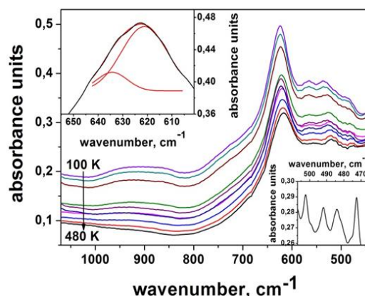
Рис. 1. ИК спектр \text{Bi}_2(\text{Sn}_{0.7}\text{Fe}_{0.3})_2\text{O}_7/\text{Bi}_2\text{Fe}_4\text{O}_9 . На вставке слева показано расщепление моды в области частот 590\text{--}680\text{ см}^{-1} . На вставке справа показана мода в области частот w=470\text{--}510\text{ см}^{-1}
