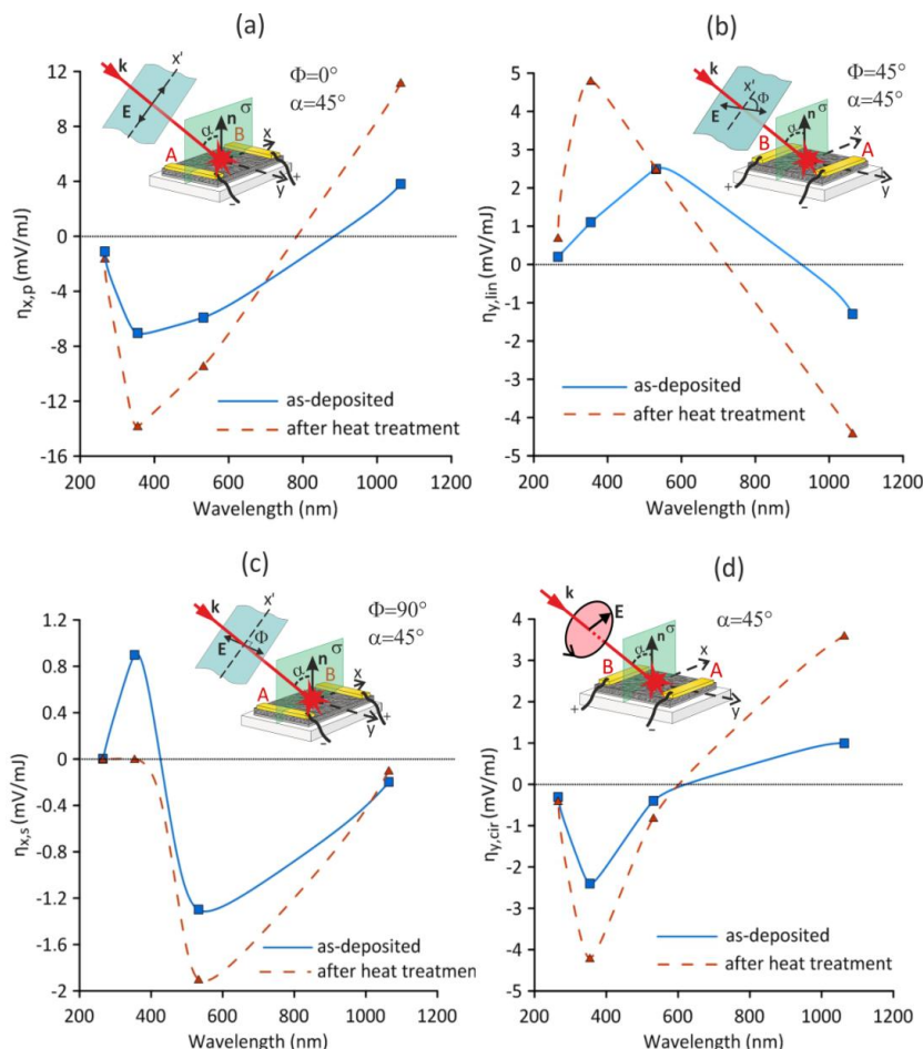
Рис. 1. Коэффициенты преобразования света в продольную фото-ЭДС при p - и s -поляризациях (а, с) и в поперечную фото-ЭДС при линейной ( \Phi = 45^\circ ) (b) и циркулярной (d) поляризациях для пленки Se(15 мг)/Cu(5 мг). Синие (квадратные) и красные (треугольные) точки соответствуют экспериментальным данным, полученным для пленок до и после их термической обработки соответственно. Во вставках показаны соответствующие схемы измерения продольной и поперечной фото-ЭДС, где А и В - измерительные электроды, прикрепленные к пленке, лежащей в плоскости x - y
