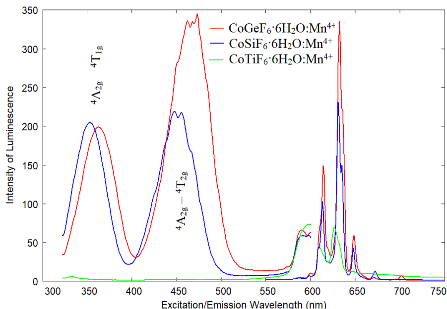
Рисунок 1. Спектры люминесценции (справа) и спектры возбуждения люминесценции (слева) кристаллов \text{CoAF}_6 \cdot 6\text{H}_2\text{O}:\text{Mn}^{4+} ( A = \text{Si}, \text{Ge}, \text{Ti} ), измеренные в 90-градусной геометрии.
