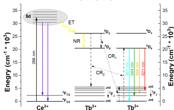
Рис. 2. Диаграмма уровней энергии системы Ce^{3+}/Tb^{3+}
