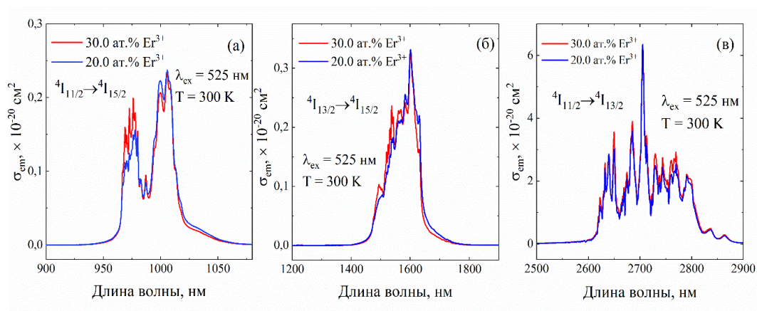
Рис. 1. Сечения вынужденного излучения кристаллов \text{BaY}_{1.8}\text{Lu}_{0.2}\text{F}_8:\text{Er}^{3+}
