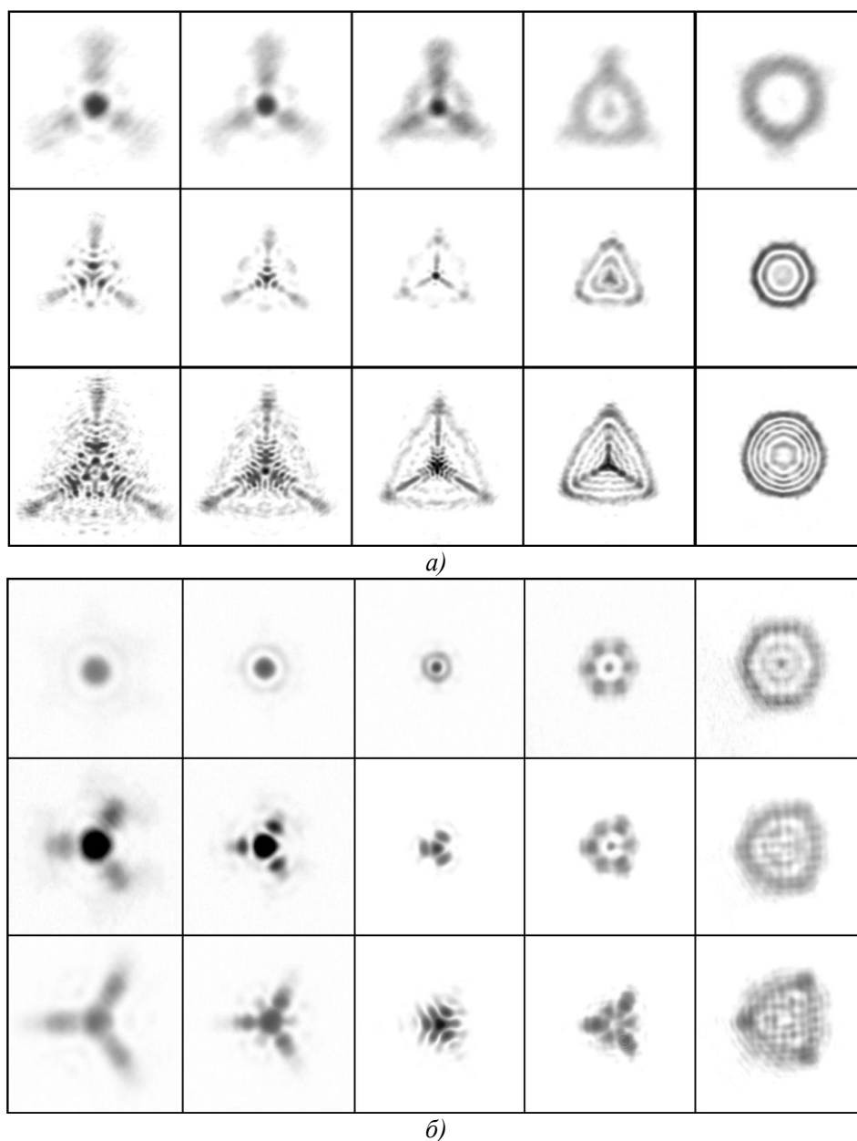
Рис. 1. Экспериментально полученные распределения интенсивности (негативы) три-Эйри (а) и три-Пирси (б) световых полей с различными параметрами смещения
