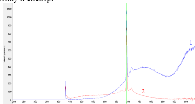
Рис. 2. Спектр послесвечения в интервале \sim (0,1 - 1) сек (1), и спектр стационарной люминесценции при непрерывном возбуждении излучением с длиной волны 405 нм (2, уменьшено в \sim 100 раз).
