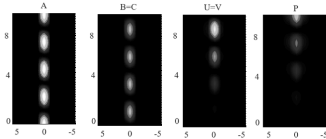
Рис. 3 Пространственное распределение интенсивности света в массивах решетки в зависимости от координаты x при накачке в торец a_0 при различных значениях констант: а) \alpha = 0.9, \beta = 0.9 \kappa = 0.01 .
