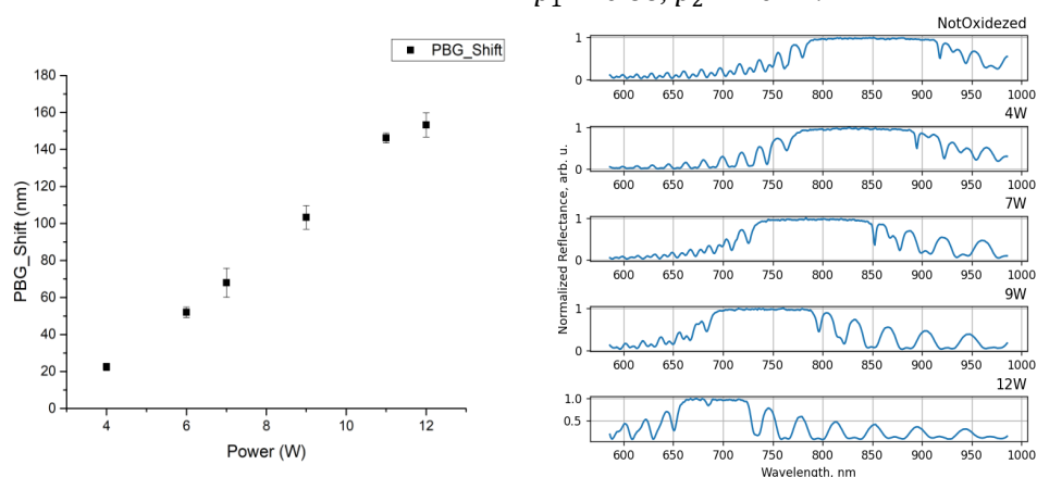
Рис. 1. (а) – сдвиг ФЗЗ фотонного кристалла в зависимости от мощности лазерного излучения, воздействию которого он подвергся. (б) – спектры отражения фотонных кристаллов для различных значений мощности лазерного излучения
