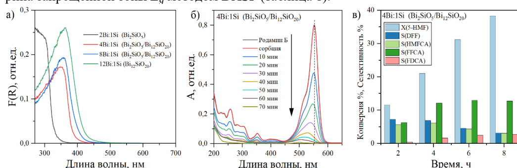
Рис. 1. Спектры поглощения образцов (а), результаты фоторазложения Родамина Б (б) и селективного фотоокисления 5-HMF (в) в присутствии катализатора 4Bi:1Si
