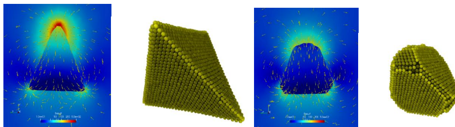
Рисунок. Локальное распределение поля вокруг идеального и деградировавшего Au нанотетраэдра на длине волны плазмонного резонанса при исчезновении острых кромок. Поляризация направлена от вершины до середины противоположной грани. Внизу – эволюция формы нанотетраэдров (максимальный размер по высоте 11 нм) при повышении температуры - от исходного состояния при комнатной температуре до 400°C (пакеты LAMPPS и Comsol Multiphysics).
