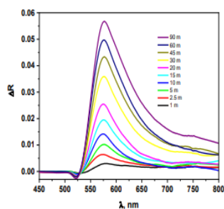
Рис.1. Изменение во времени дефектного поглощения в CsPbBr 3 , легированном Ag (0,44 ат.%), вызванное облучением при \lambda=436 нм: разница в спектрах диффузного отражения при разных временах засветки Hg лампой.
