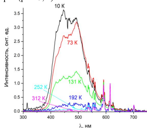
Рисунок 3. Спектр люминесценции образца \text{LiGdF}_4 :Eu 3+ (1 ат.%) в диапазоне температур 10-290K, при возбуждении 274нм ( \text{Gd}^{3+} ).
