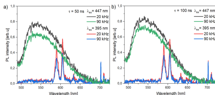
Рис. 2. Спектры фотолюминесценции ФГК с поверхностью, обработанной лазерным излучением с частотой следования импульсов 20 и 90 кГц: a – 50 нс, b – 100 нс.
