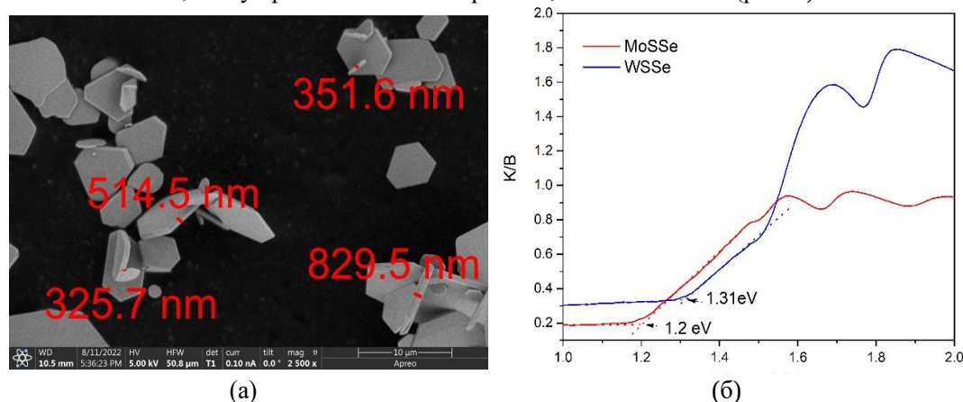
Рис. 1. SEM-изображение пластин MoSSe (а), зависимость функции Кубелки-Мунка от энергии фотона (б).
