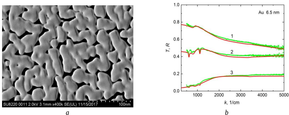
Рис. 1. а) Электронно-микроскопическое изображение слоя золота толщиной 5 нм. б) Коэффициенты отражения при падении излучения со стороны слоя золота толщиной 6,5 нм (1) и со стороны кремниевой подложки (2), а также коэффициент пропускания (3) для структуры №1 в зависимости от волнового числа. Точки – эксперимент, линии – расчет ( R_{S0}=9\text{ Ом}/\Omega , \tau=8 фс, p=0,79 , g=0,68 ).
