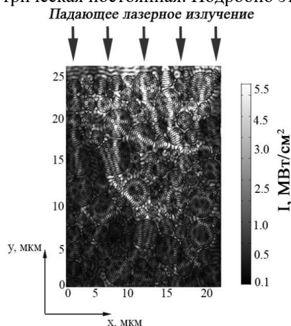
Рис. 1. Распределение интенсивности излучения волоконного лазера рассеянного при прессованном порошке из \text{Y}_2\text{O}_3 . Интенсивность падающего излучения 0.46 \text{ MBt/cm}^2
