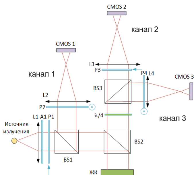
Рис. 1. Схема матричного поляриметра
