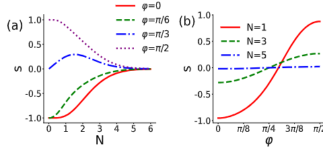
Рис.1 Зависимость коэффициента перекрытия s от числа колебаний в импульсе N для разных значений начальной фазы \varphi (a) и от \varphi для разных значений N (b).
