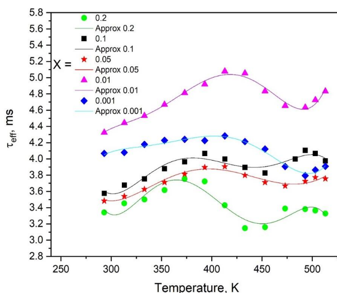
Рис.1. Эффективные времена затухания люминесценции ионов \text{Tb}^{3+} в зависимости от температуры. Детектирование производилось на длине волны 541 нм соответствующей ^5\text{D}_4 - ^7\text{F}_5 излучательному переходу ионов \text{Tb}^{3+}
