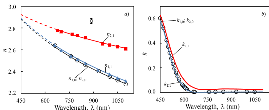
Рис. 1. Дисперсионные зависимости показателя преломления n (a) и коэффициента экстинкции k (b) плёнок \text{Ge}_{10}\text{Se}_{90} до ( n_{1,0} , k_{1,0} ; n_{2,0} , k_{2,0} ) (первый нижний индекс, равный 1 или 2, соответствует образцу №1 или №2, второй нижний индекс равен 0) и после их термического отжига ( n_{1,1} , k_{1,1} ; n_{2,1} , k_{2,1} ) (второй нижний индекс – 1). Температура отжига для образца №1 составляла 303 \pm 2 К, для образца №2 – 363 \pm 2 К
