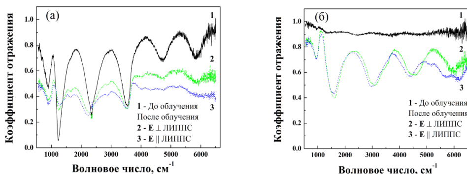
Рис. 1. Спектры отражения исходных и облученных пленок аморфного кремния толщиной 1 мкм на стеклянной подложке без напыления верхнего слоя (а) и с напыленным сверху слоем алюминия (б).
